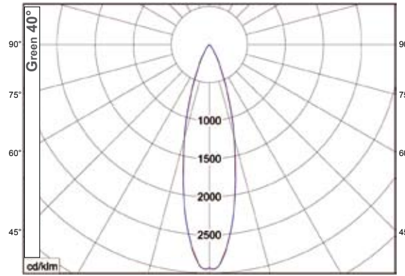
half value angle C0-C180 : 26,4° C90-C270 : 26,6°
