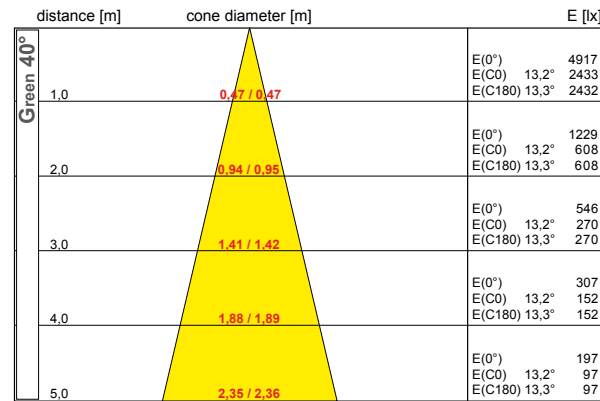
half value angle C0-180 : 26,4° C90-270 : 26,6° 24xLED, total flux: 1680,0 lm, LOR: 85%
