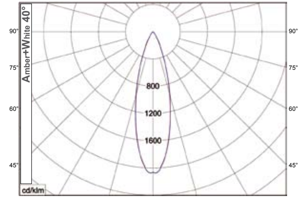
half value angle C0-C180 : 27,6° C90-C270 : 28,0°
