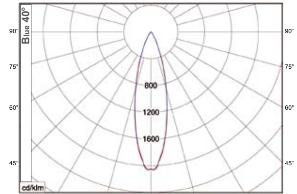
half value angle C0-C180 : 26,6° C90-C270 : 26,4°
