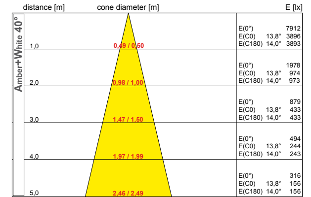
half value angle C0-180 : 27,6° C90-270 : 28,0° 54xLED, total flux: 3840,0 lm, LOR: 63%
