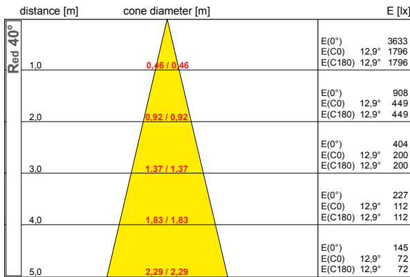
half value angle C0-180 : 25,8° C90-270 : 25,8° 30xLED, total flux: 1440,0 lm, LOR: 70%
