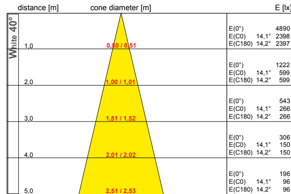
half value angle C0-180 : 28,2° C90-270 : 28,4° 24xLED, total flux: 2400,0 lm, LOR: 65%
