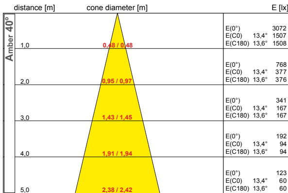
half value angle C0-180 : 26,8° C90-270 : 27,2° 30xLED, total flux: 1440,0 lm, LOR: 64%
