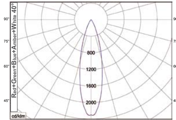
half value angle C0-C180 : 26,6° C90-C270 : 26,8°
