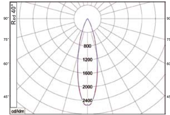
half value angle C0-C180 : 25,8° C90-C270 : 25,8°
