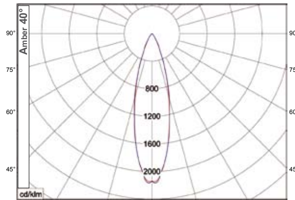
half value angle C0-C180 : 26,8° C90-C270 : 27,2°
