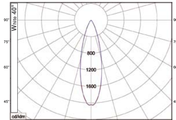
half value angle C0-C180 : 28,2° C90-C270 : 28,4°
